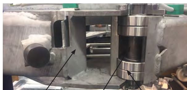
verschleißfreie Lagerbuchse
